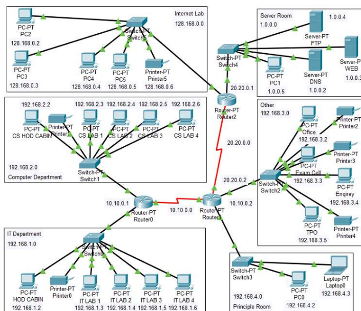
Capture d'écran Cisco Packet Tracer
